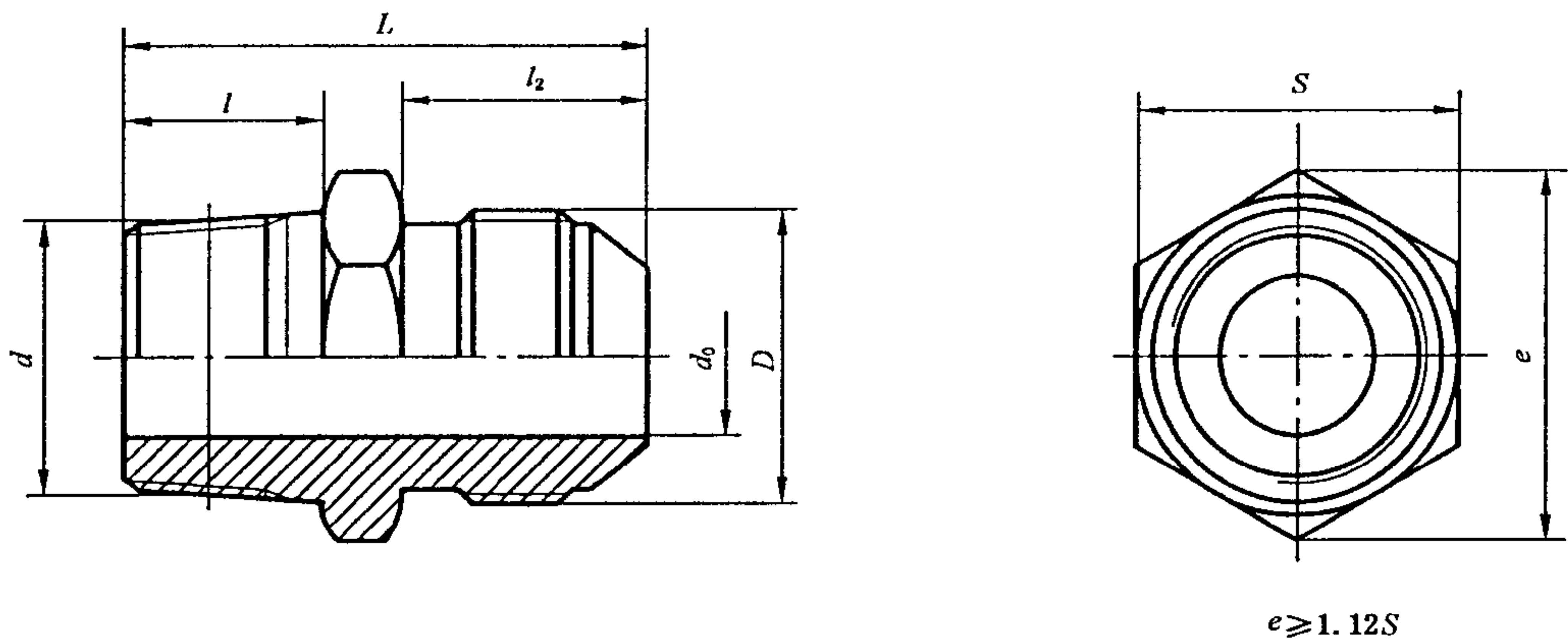
图 2 扩口式锥螺纹直通接头体
