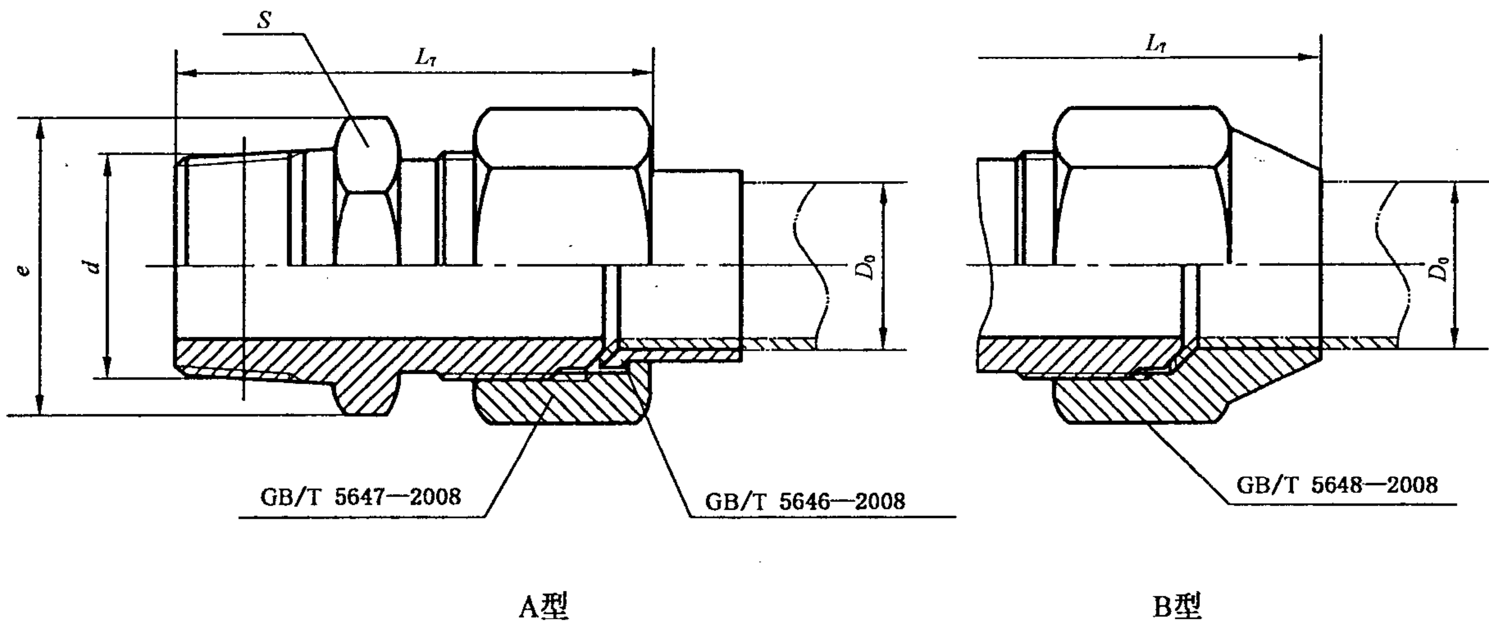
图 1 扩口式锥螺纹直通管接头
